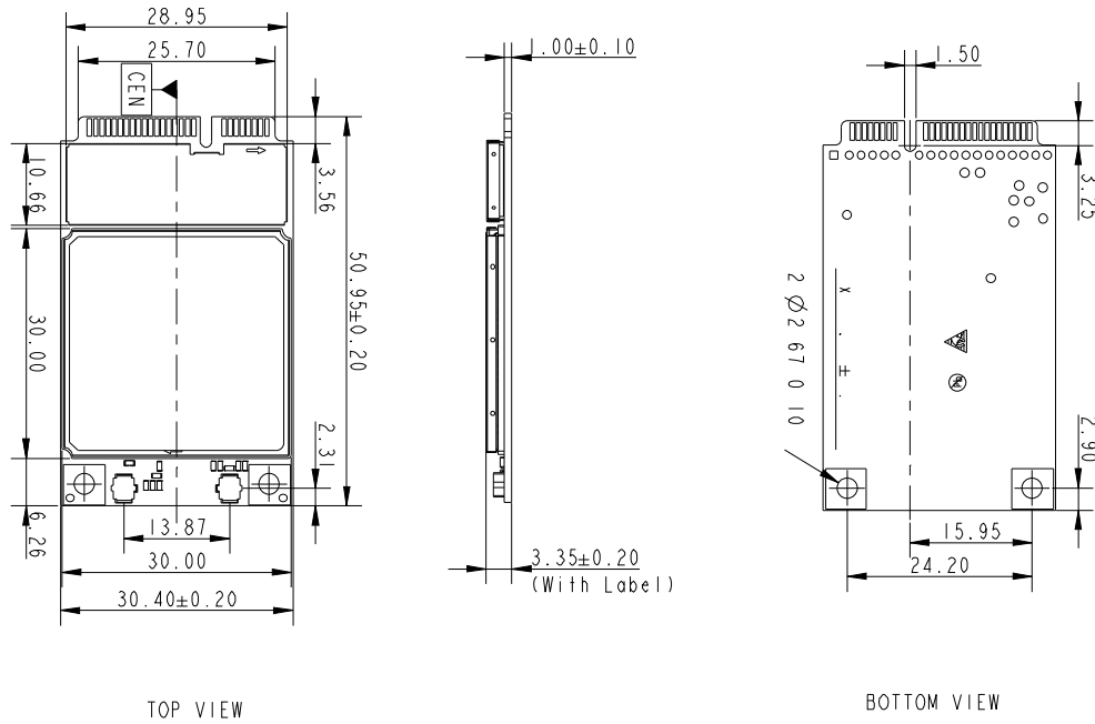
Figure 6-1 Dimensions of the ME209u-526 Mini PCIe module (unit: mm)
